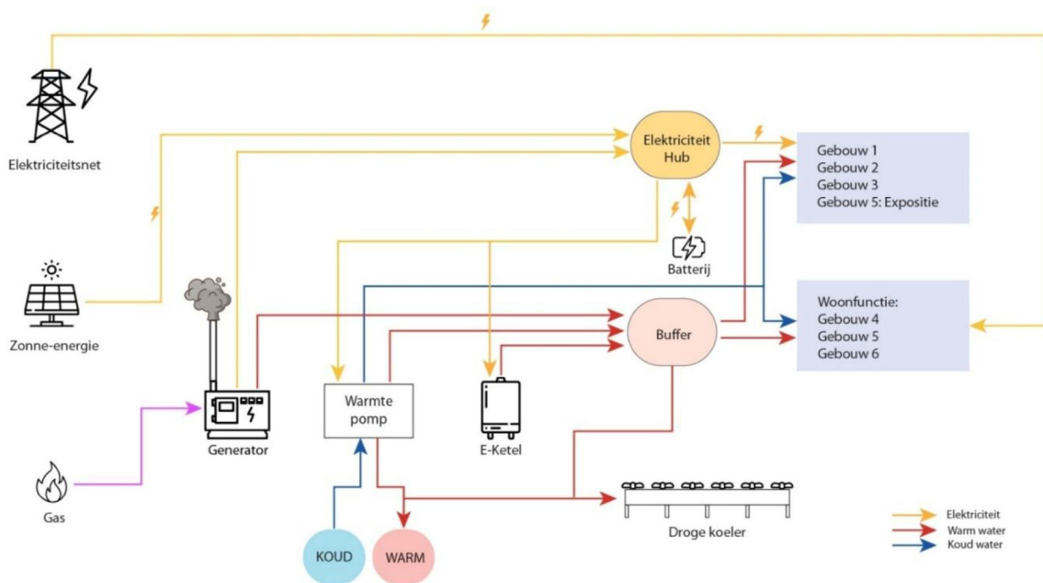
Figuur 17: Schematische weergave van voorgestelde installatieprincipe
