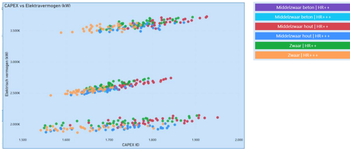
Figuur 15 : Overzicht elektrische piekvermogens per iteratie
